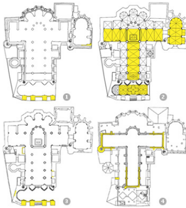
Plantas siglo XV: 1- Planta paso de ronda. 2- Planta bóvedas. 3. Planta baja. 4. Planta triforio.
