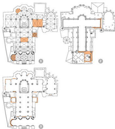
Plantas siglo XVI: 1- Planta bóvedas. 2- Planta triforio. 3. Planta baja.
